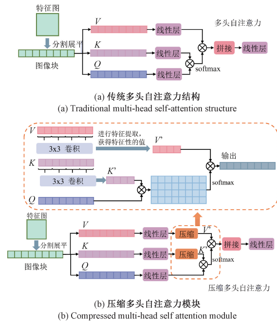
图5 传统多头自注意力结构和压缩多头自注意力模块
