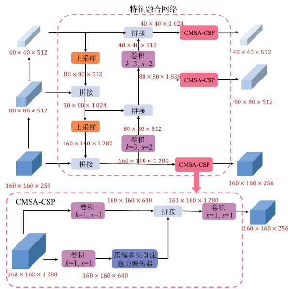
图3 特征融合网络参数
