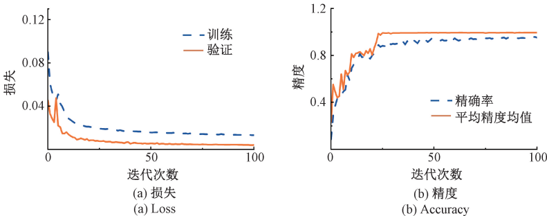
图 9 训练过程中记录的指标
