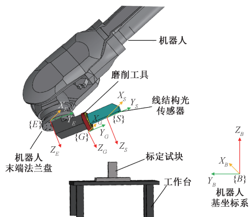
图1 系统模型
