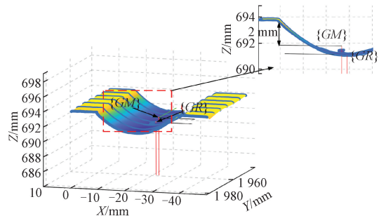
图 13 标定前理想与当前坐标系位置
