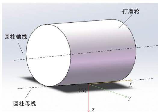
图3 打磨轮模型
