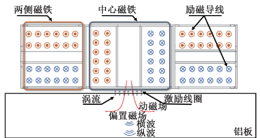
(a) EMAT激励超声波原理图
