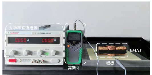
(a) 磁通密度测量实验平台
