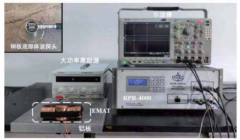
图 16 实验平台
