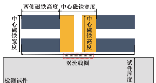
(b) 仿真几何模型
