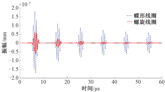
图 12 蝶形线圈与螺旋线圈试件内部横波位移图
