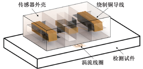
图3 海尔贝克式电磁铁 EMAT 示意图
