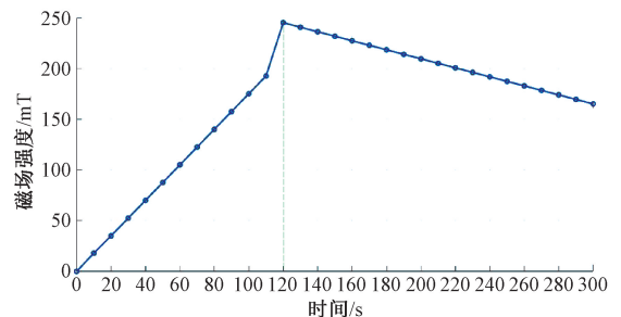
(b) 磁通密度随通电时间的变化曲线
