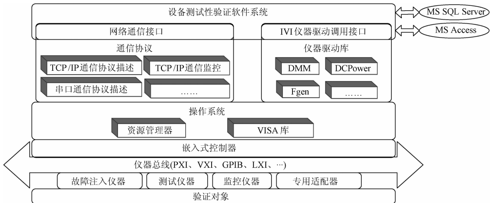
图 5 测试性验证与评估平台的技术体系结构
