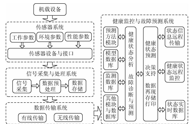
图 3 军用飞机 PHM 系统
