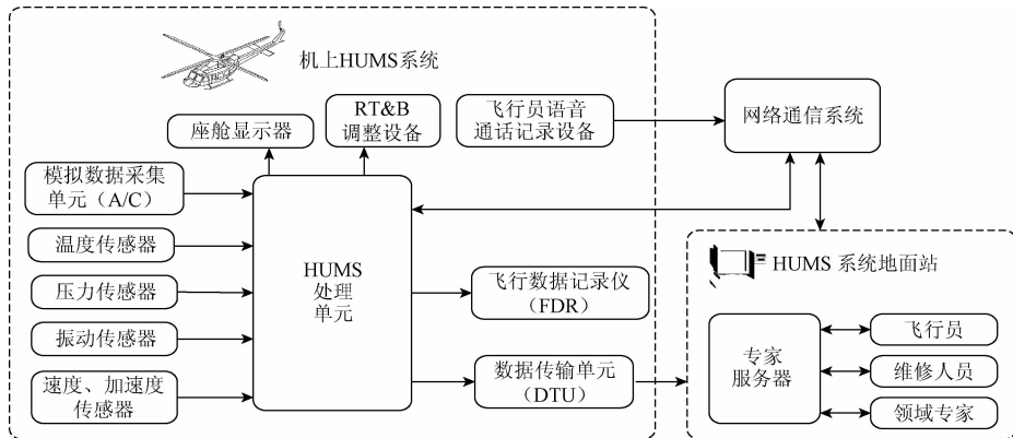
图 1 先进直升机 HUMS 系统结构
