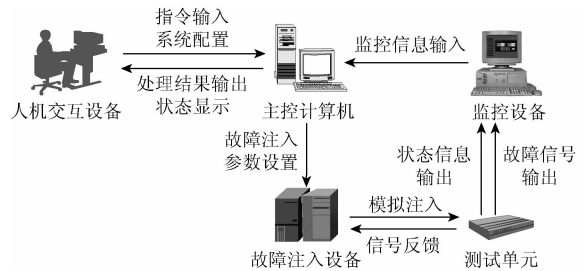
图 4 测试性验证试验的实施过程
