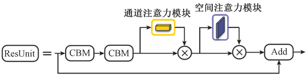
图 5 添加 CBAM 的 ResUnit 结构
